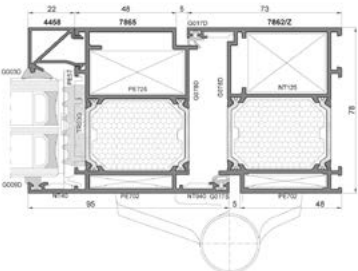
Przekrój drzwi Procural PE78N HI
