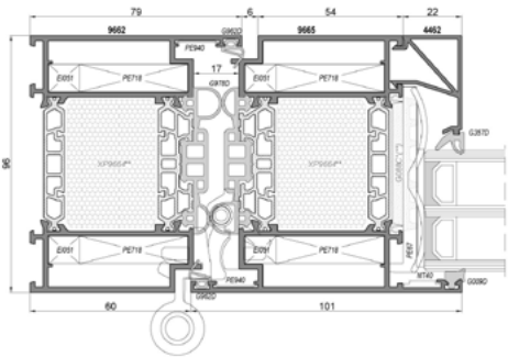
Przekrój drzwi Procural PE96HI
