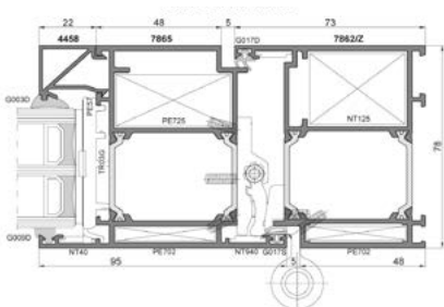
Przekrój drzwi Procural PE78N
