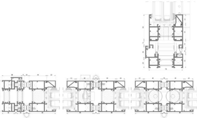
Przekrój drzwi PROCURAL PE78 FOLD
