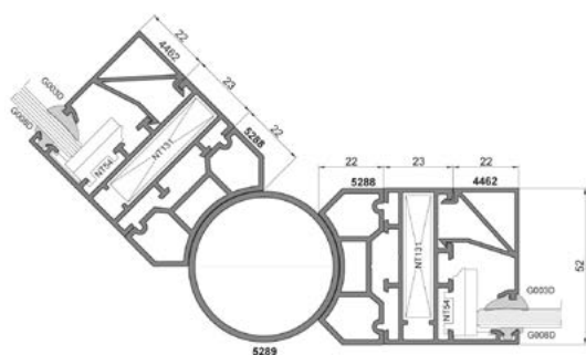
Przekrój ścianki Procural PE50
