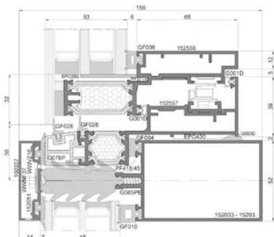
Przekrój Procural PF152HI
