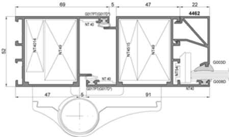
Przekrój drzwi Procural PE50
