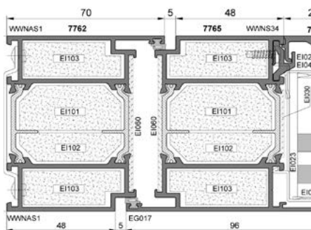
Przekrój PROCURAL PE78EI DESIGN LINE kl. EI60
