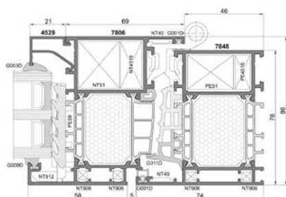
Przekrój okno Procural PE78N HI
