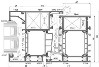
Przekrój okna Procural PE78N
