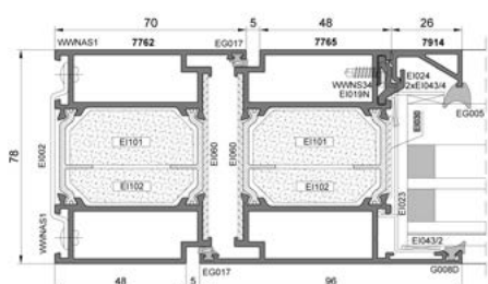
Przekrój PE78EI DESIGN LINE kl. EI30
