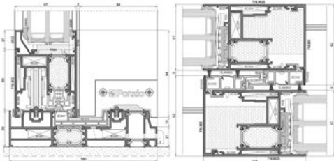
Przekrój okna podnoszono-przesuwnego Procural SL1600TT HI
