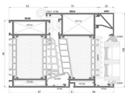
Przekrój okno Procural PE96
